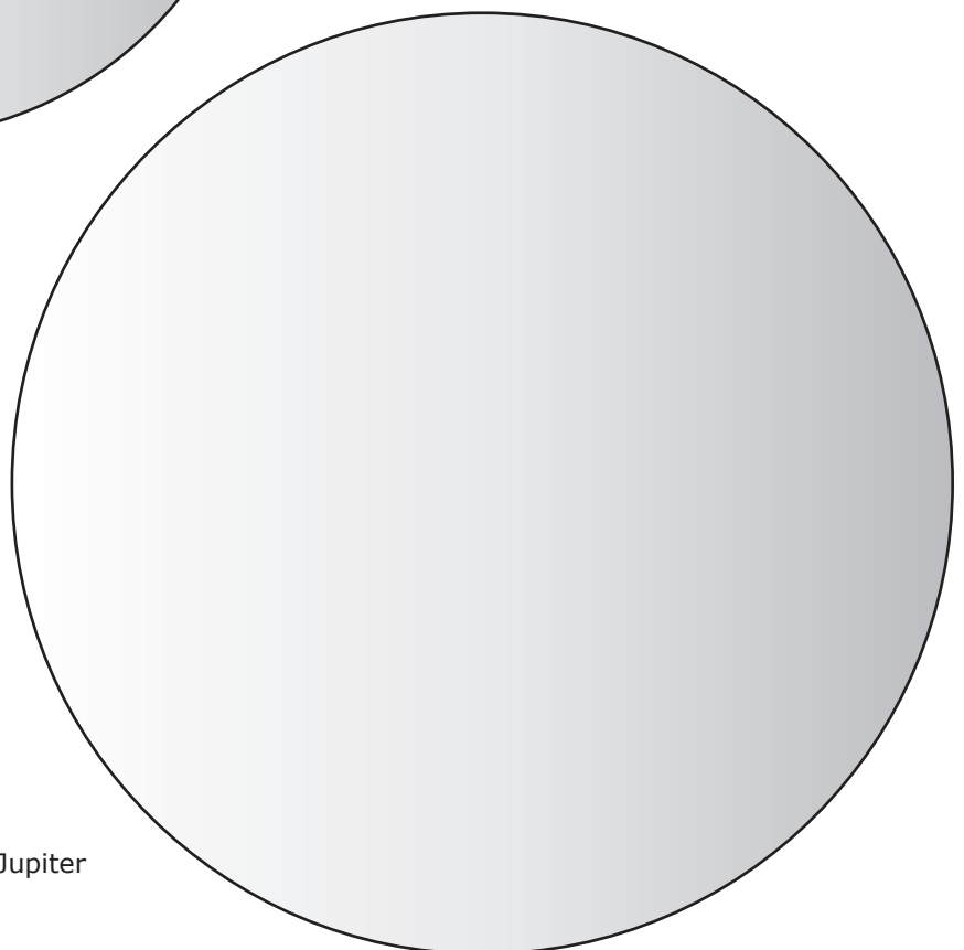
Uranus
