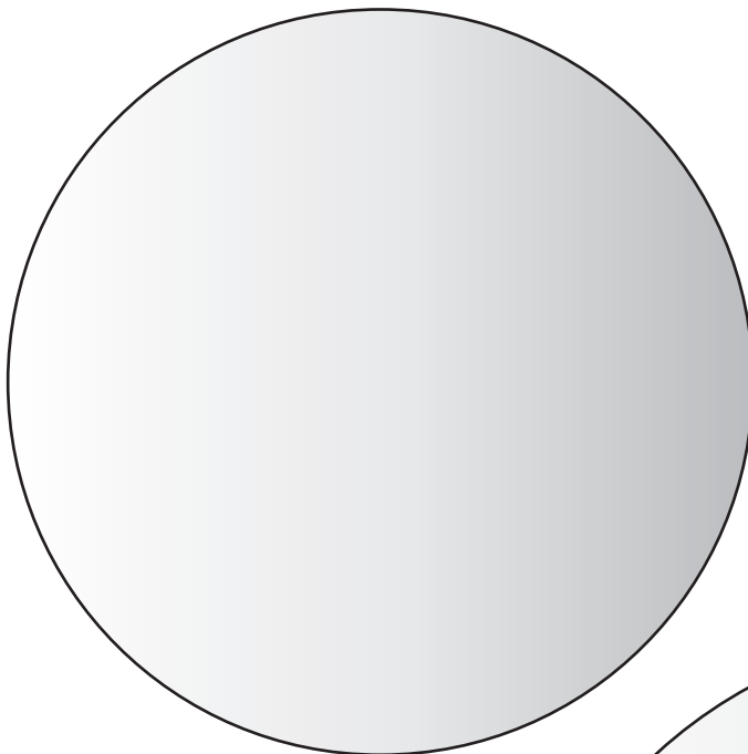
Saturnus
