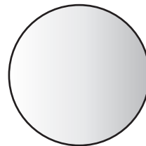
Neptunus
