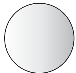
Uranus
